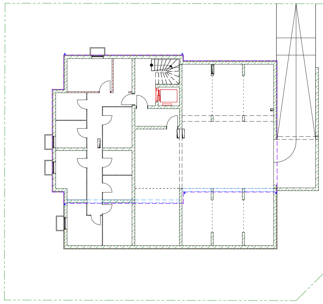
GRUNDRISS - UNTERGESCHOSS M 1 : 200
