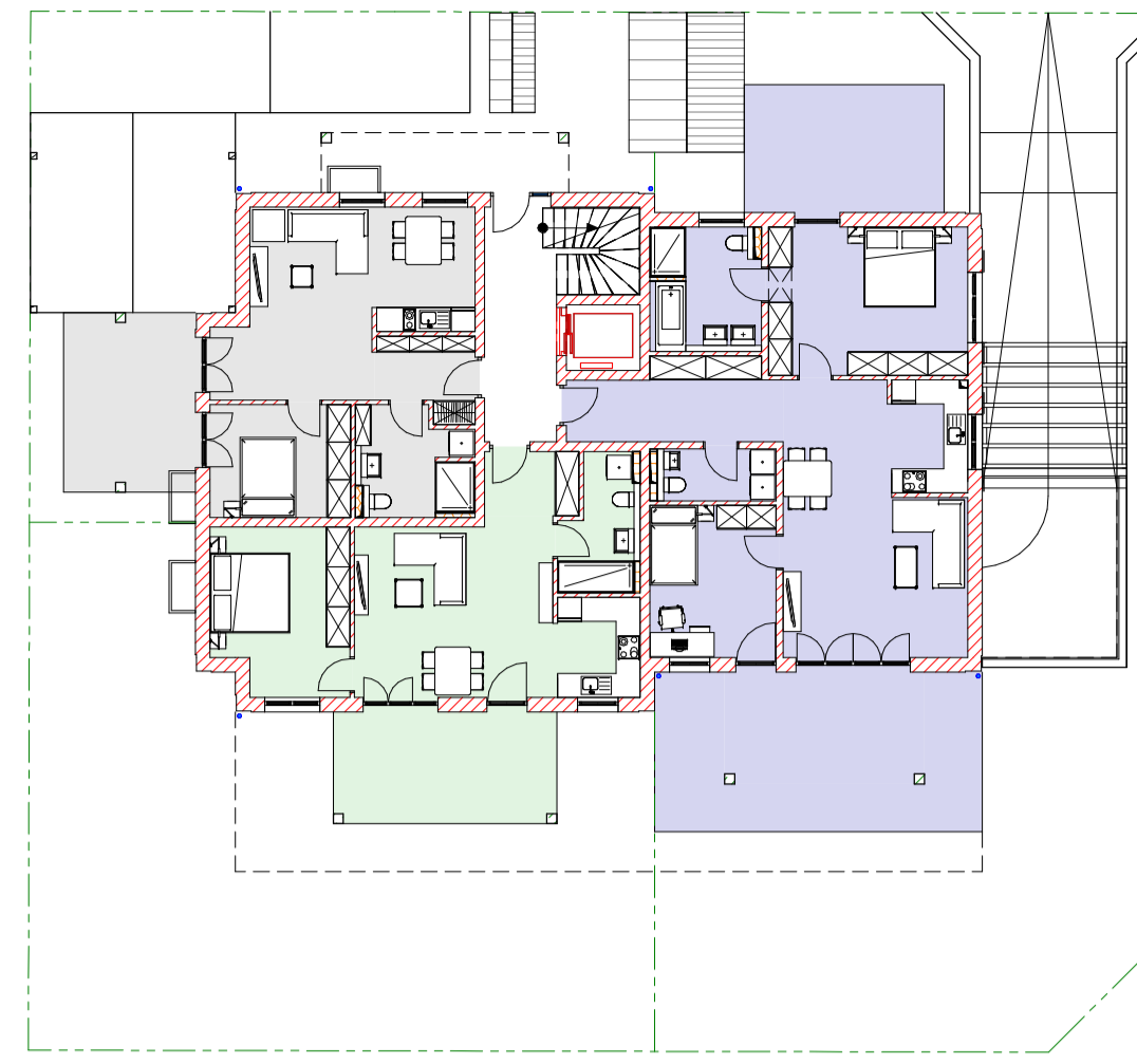
GRUNDRISS - ERDGESCHOSS M 1 : 200
