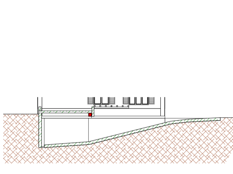
SYSTEMSCHNITT 4 M 1 : 200
