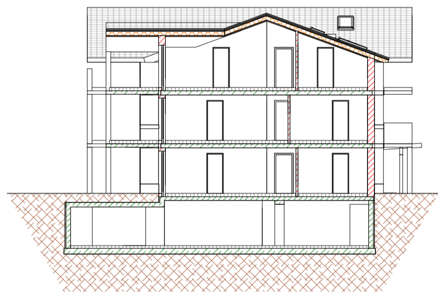
SYSTEMSCHNITT 1 M 1 : 200
