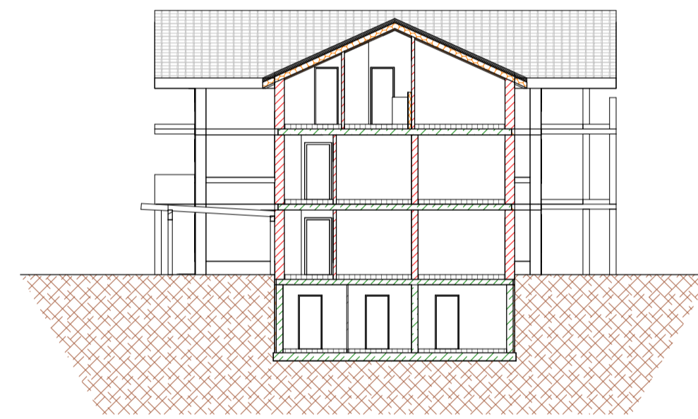
SYSTEMSCHNITT 3 M 1 : 200
