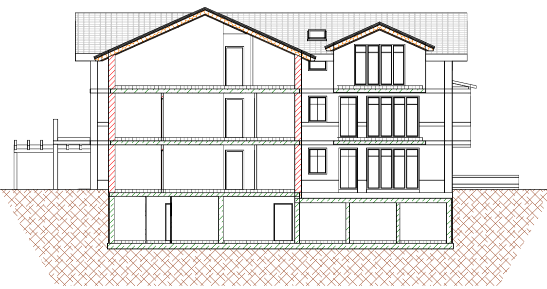
SYSTEMSCHNITT 2 M 1 : 200
